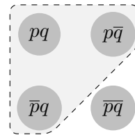
Figure 6.39: [\neg q \rightarrow \neg p]^-
