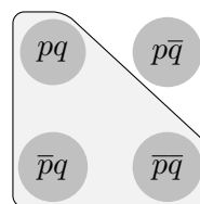
Figure 3.8: \neg q \rightarrow \neg p
