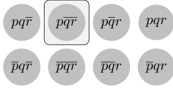
Figure 6.42: (\neg p \rightarrow_m (\neg q \rightarrow_m r)) \wedge (\neg(\neg q \rightarrow_m r))
