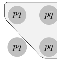
Figure 7.12: \neg p \rightarrow \neg q
