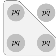
Figure 6.35: \neg q \rightarrow_m \neg p
